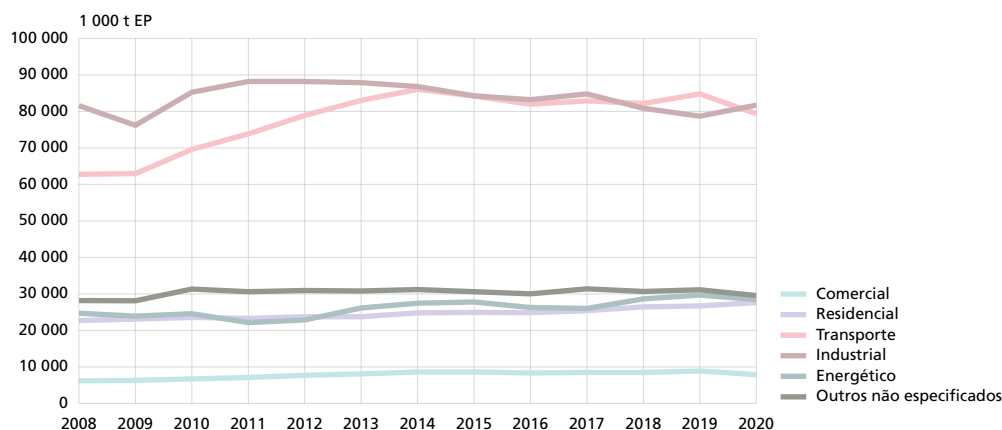
Gráfico 4.3.1 Evolução do consumo final de energia, por setor - 2008-2020
