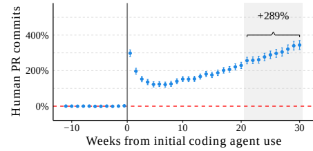
(d) 0.1% winsorization: Pooled Sync
