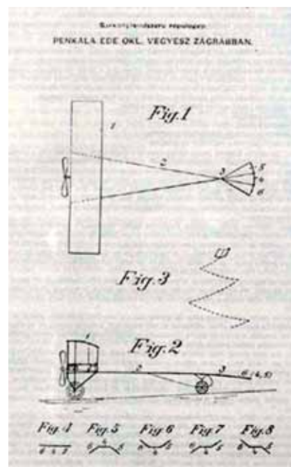
Nacrt zrakoplova Slavoljuba Penkale
