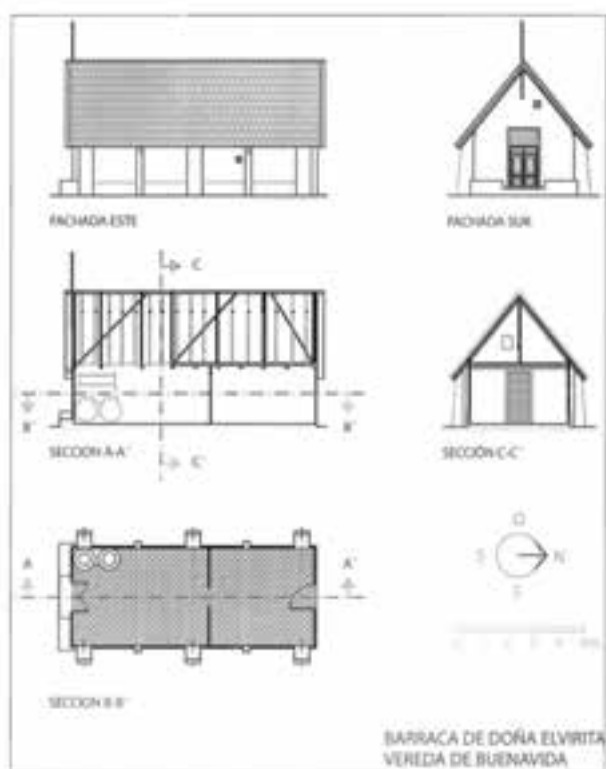
Planta, alzado y sección de una barraca prototípica de la huerta bajosegureña. Según Antonio Rodríguez Cases.
