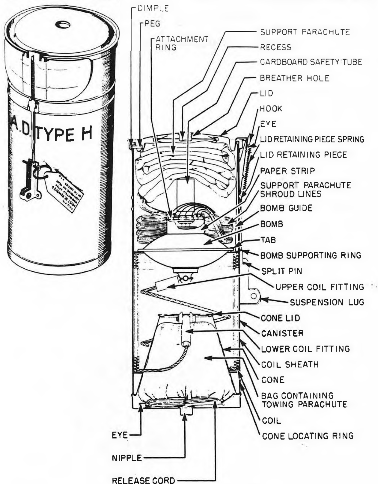
Figure 63—Type H., A.D. Apparatus Mk II
