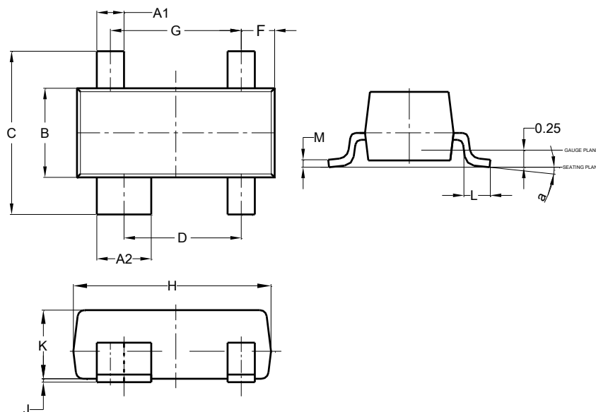
SOT143
