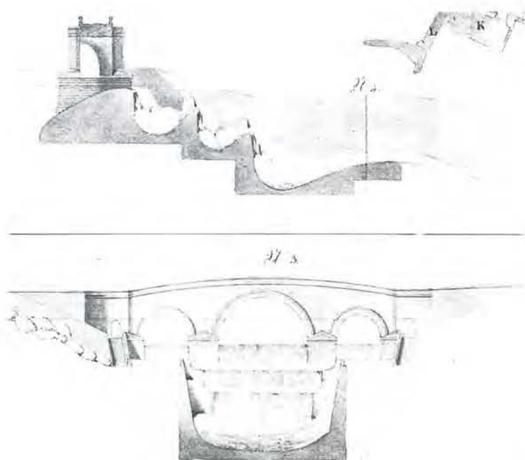
Progetto Kessels per una nuova chiusa e ponte.
