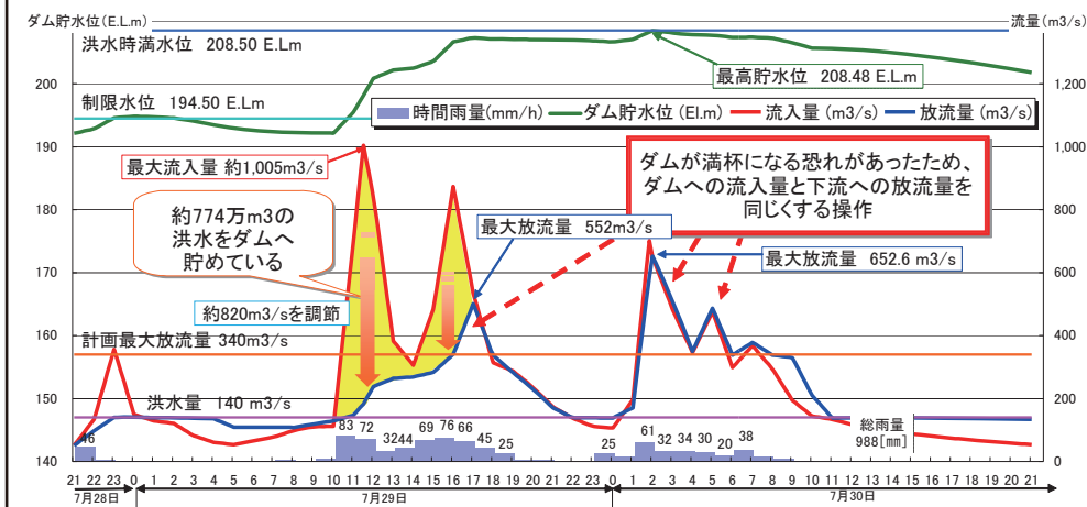
信濃川水系五十嵐川の笠堀ダムでは、最大約774万m 3 の洪水を貯留。またダム地点への最大流入量約1,005m 3 /sを約820m 3 /s調節し、下流の氾濫量の軽減に寄与。
