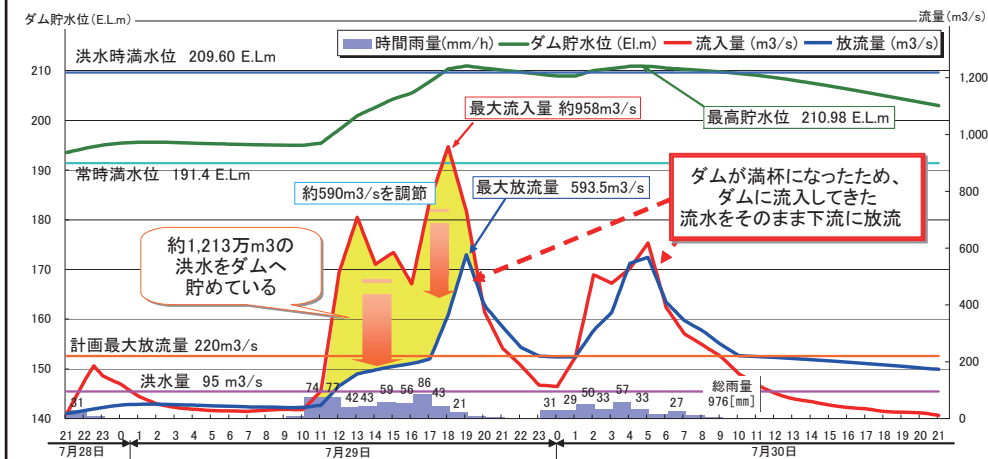
信濃川水系五十嵐川の大谷ダムでは最大約1,213万m 3 の洪水を貯留。また、ダム地点への最大流入量約958m 3 /sを590m 3 /s調節し、下流の氾濫量の軽減に寄与。
