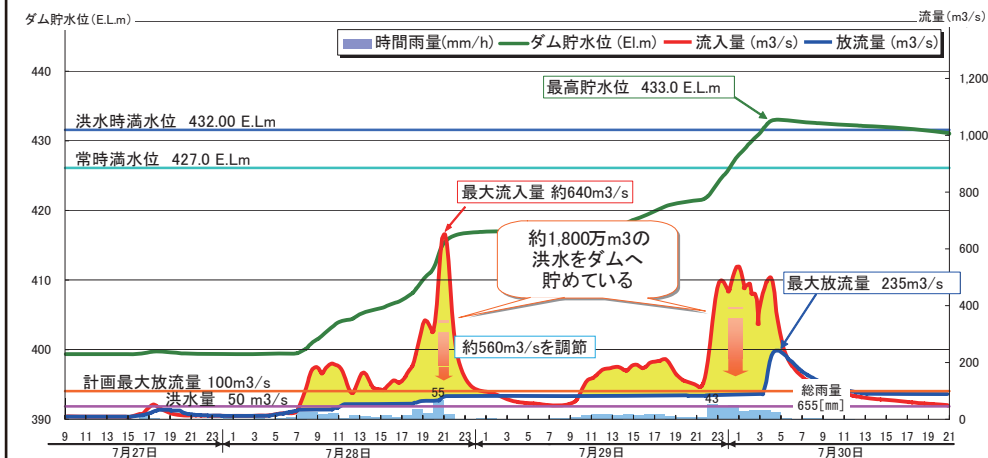
信濃川水系三国川の三国川ダムでは最大約1,800万m 3 の洪水を貯留。また、ダム地点への最大流入量約640m 3 /sを約560m 3 /s調節し、下流の水位低下に寄与。
