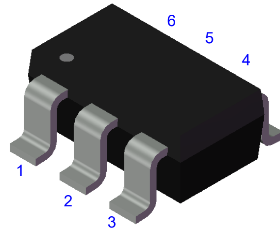
SOT26 PACKAGE
